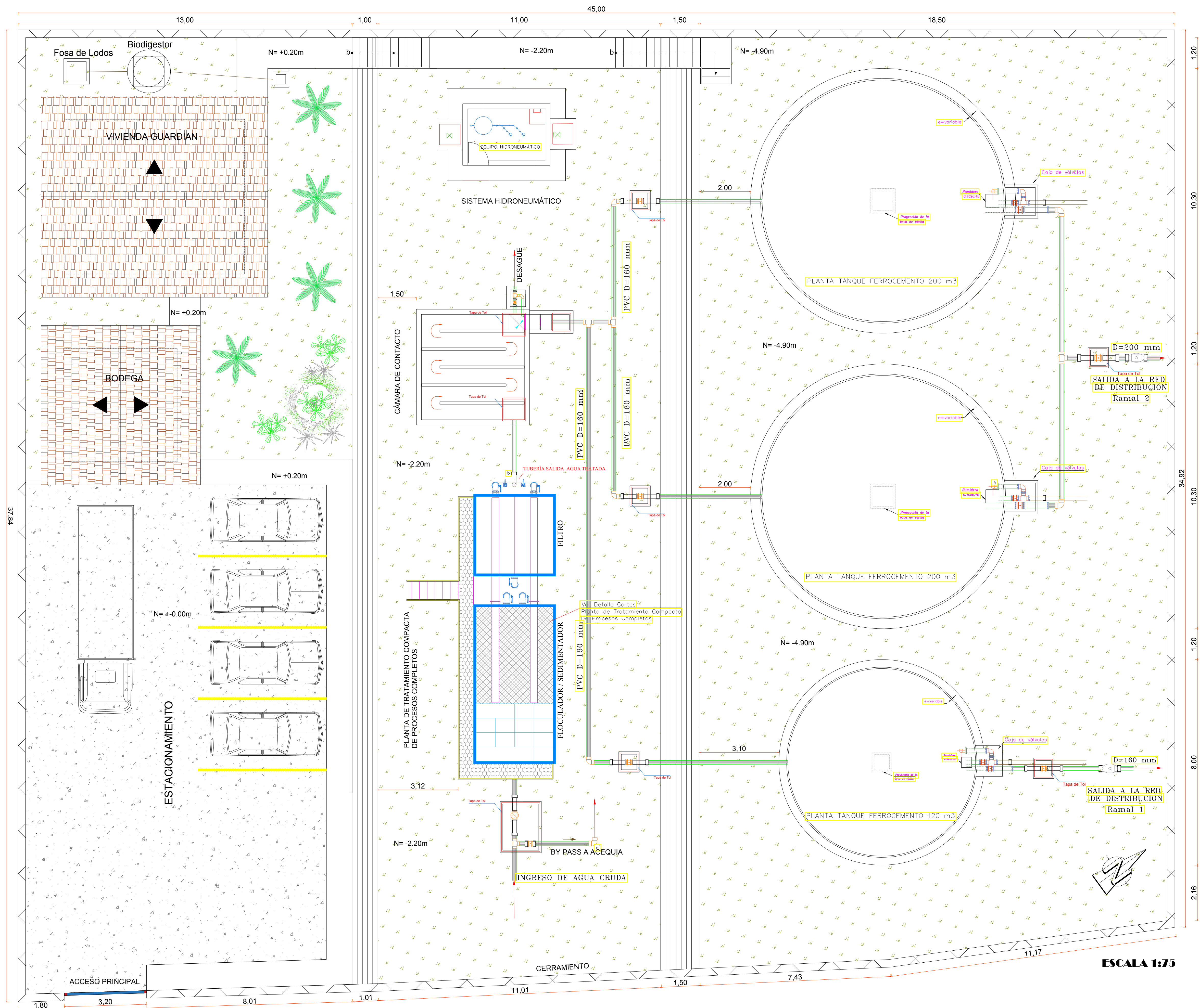
DETALLE PLANTA DE TRATAMIENTO
